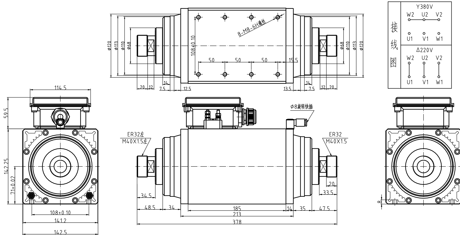
GDF71-18Z/4.5S外形图
